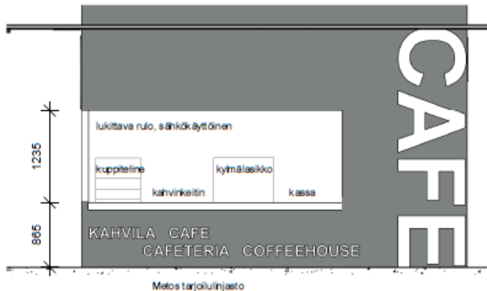
Projektio C4, tarjotinlinjasto 1 : 50
